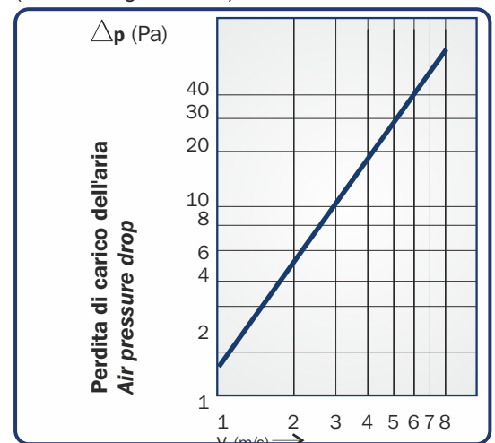
(Altezza/height mm 65)
